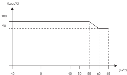
115V Load Loss(%)@Temperature(°C)
